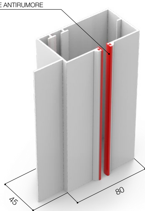
Guida con alette - cod. 964
