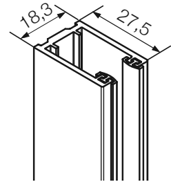
Guida fissa FD cod. 945
