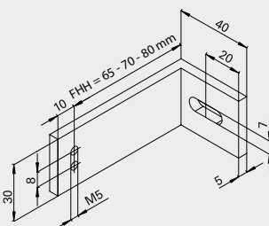
Squadretta per guide a L cod. tipo 1
