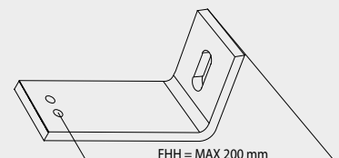
Squadretta per guide a gomito cod. tipo 5
