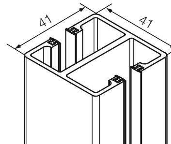
Supporto centrale cod. 934
