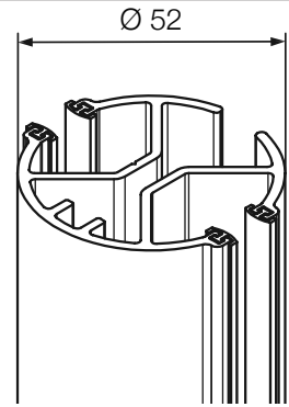
Guida doppia FDR cod. 955
