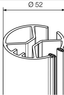
Guida semplice FER cod. 944
