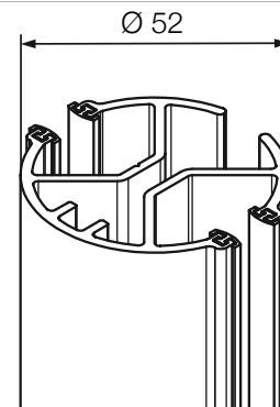
Guida doppia FDR cod. 955
