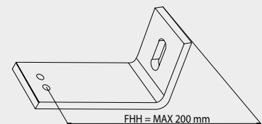
Squadretta per guide a gomito in ghisa cod. tipo 5
