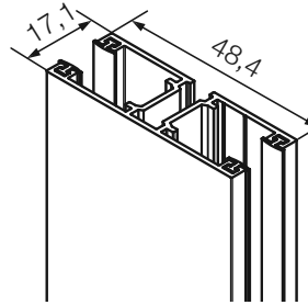
Guida doppia FD cod. 954
