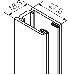
Guida fissa FD cod. 945
