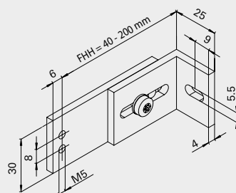
Squadretta per guide FEH cod. tipo 3
